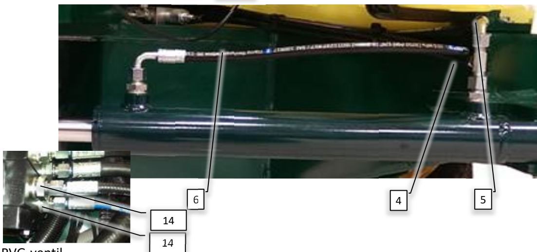
PVG-ventil
