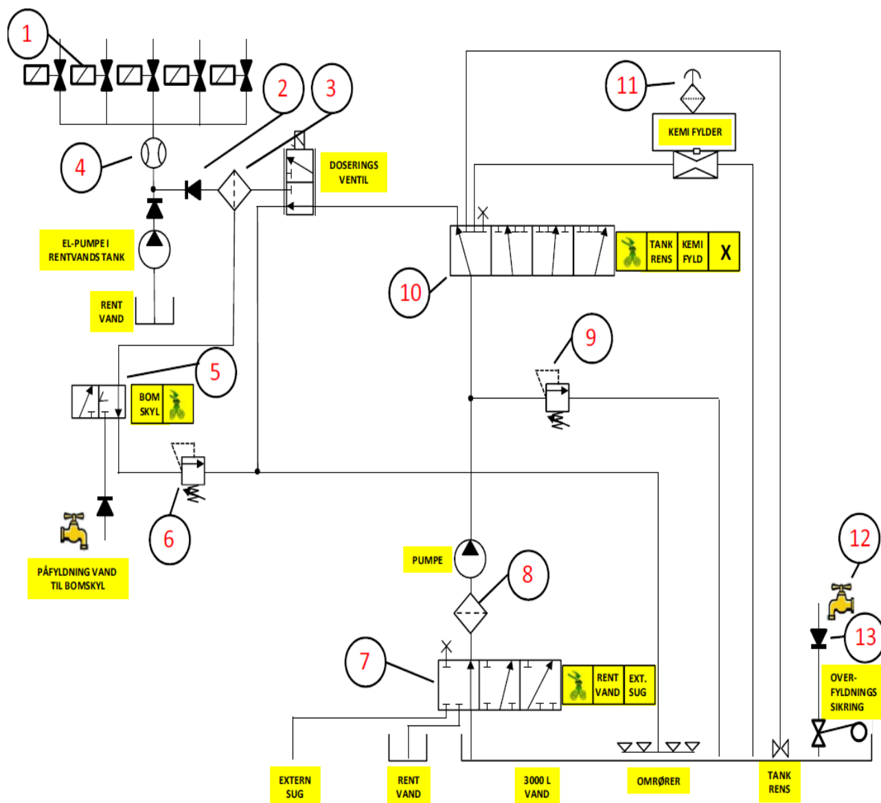
Diagram 1: Sprøjtens funktioner
